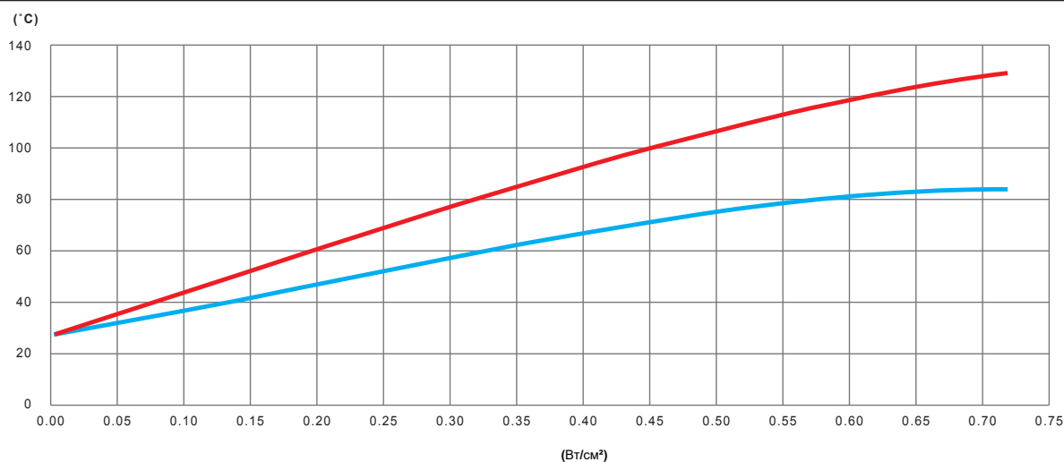
Изменение в зависимости от мощности в Вт/см² силиконовой нагревательной ленты и температуры стенки трубы из PVC, заполненной нециркулирующей водой, без теплоизоляции.
