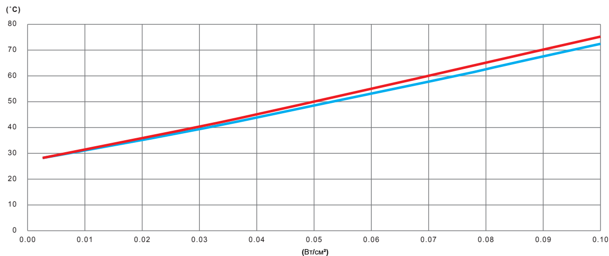
Изменение в зависимости от мощности в Вт/см² силиконовой нагревательной ленты и температуры стенки пустой трубы из PVC, теплоизолированной 20 мм пены PVC-NBR
